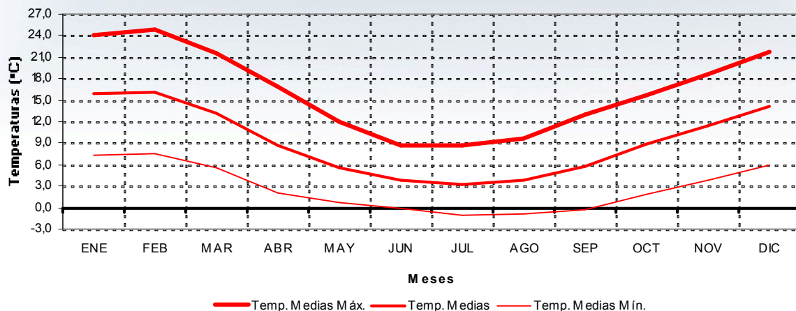
TEMPERATURAS MÁXIMAS, MEDIAS Y MÍNIMAS - PROMEDIO 2001 - 2010
